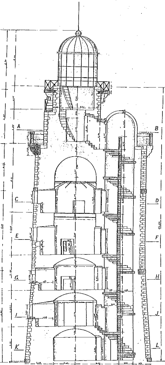
COUPE VERTICALE.
