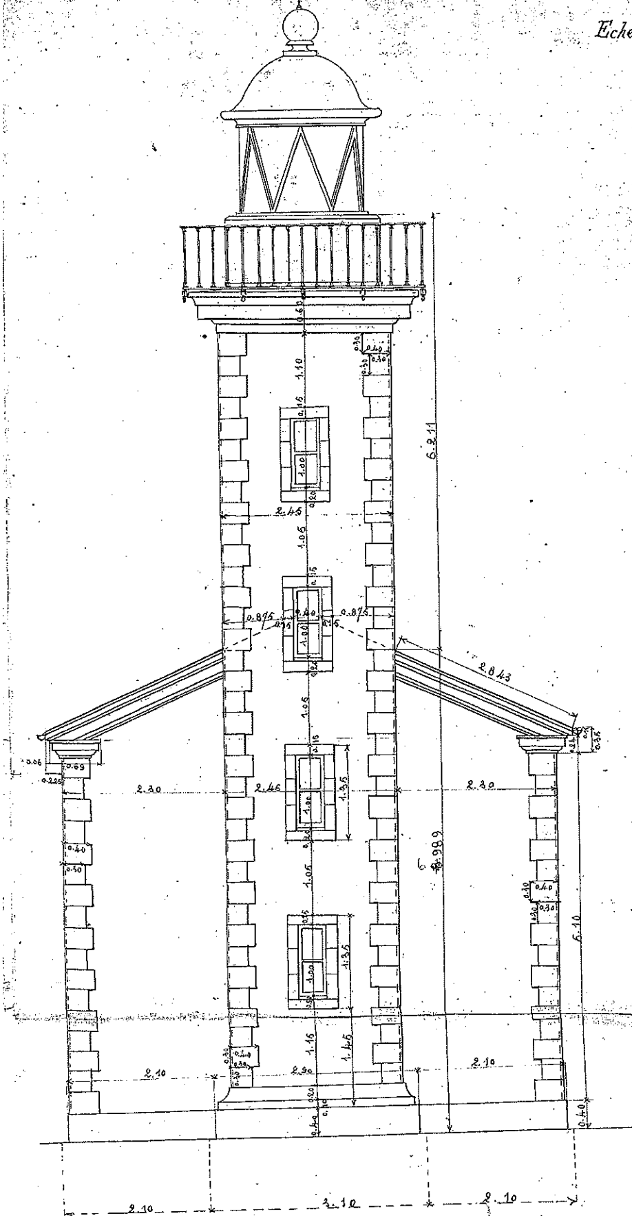
Elevation de la tour et du Pignon sud.
