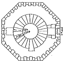
COUPE EF
