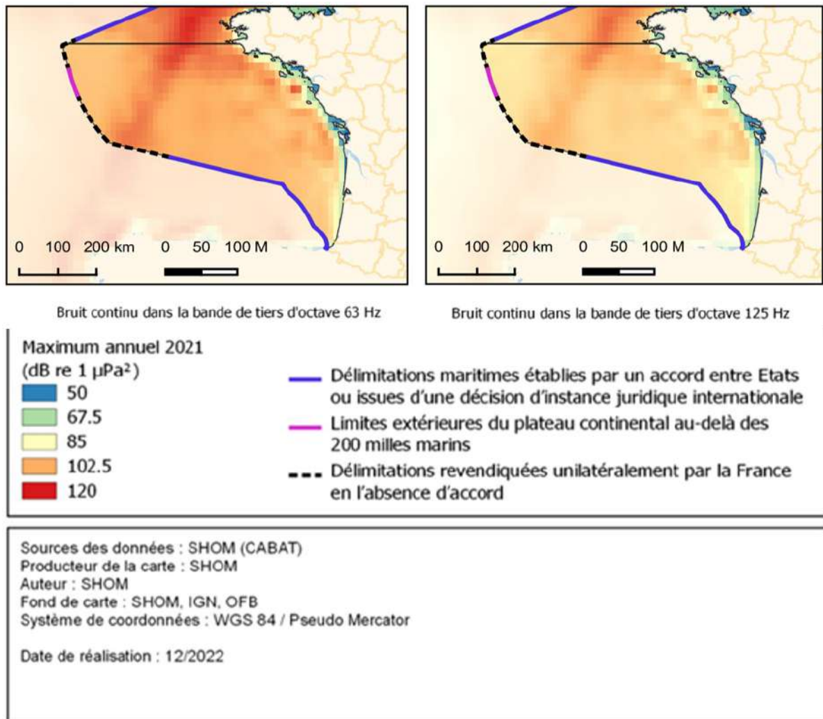
Figure 9 : Maximum annuel du bruit continu dans les bandes de fréquence (dites bandes de tiers d'octave) 63 Hz (gauche) et 125 Hz (droite) pour l'année 2021 (dB re 1 \mu\text{Pa}^2 ) dans la sous-région marine Golfe de Gascogne.
