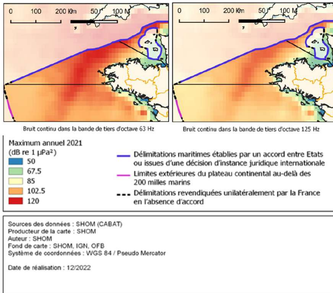
Figure 4 : Maximum annuel du bruit continu dans les bandes de fréquences (dites bandes de tiers d'octave) 63 Hz (gauche) et 125 Hz (droite) pour l'année 2021 (dB re 1 \mu\text{Pa}^2 ) dans la sous-région marine Mers Celtiques.
