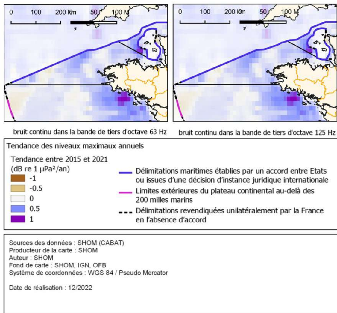
Figure 5 : Tendence, entre 2015 et 2021, des niveaux maximaux annuels [bruit continu dans les bandes de fréquences (dites de tiers d'octave) 63 Hz (gauche) et 125 Hz (droite)] pour la sous-région marine Mers Celtiques.
