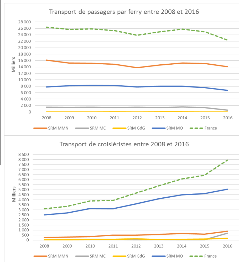
Figure 2 : Evolution du nombre de passagers (croisiéristes et par ferry) par sous-région marine et à l'échelle nationale entre 2008 et 2016 (source SoeS/SDDES)
