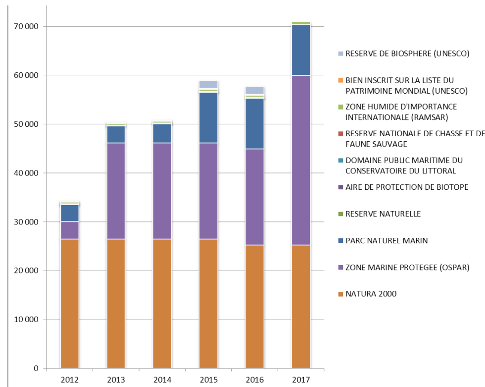
Figure 5: Évolution de la surface (en km²) par type de protection à l'échelle de la façade Atlantique (au sens de la zone de compétences de la préfecture maritime) (Source : AFB, 2017)
