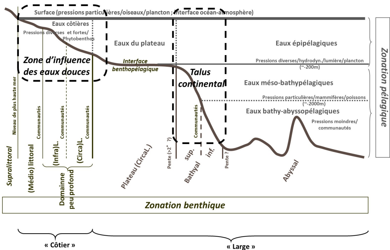
Figure : Schéma des composantes principales des habitats benthiques et pélagiques, selon un gradient côte-large et un zonage verticale. Le talus continental et la limite (schématisée) d'influence des apports par les eaux douces sont entourés par des tirets noirs pour souligner les enjeux spécifiques à ces secteurs.
