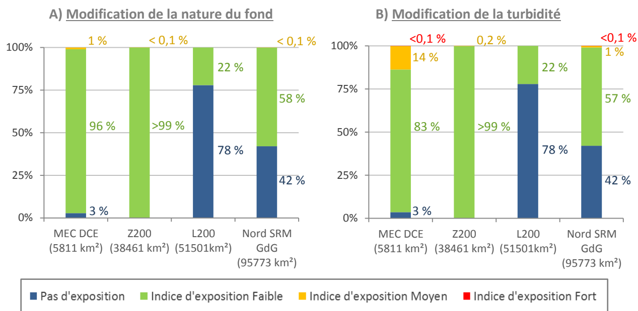
Figure 10 : Répartition (en % de surface) de la modification permanente de la nature du fond (A) et de la turbidité (B) pour chaque UMR et pour la subdivision Nord de la SRM GdG selon quatre niveaux d'indice d'exposition. La superficie indiquée entre parenthèse représente la superficie totale de l'UMR ou de la subdivision Nord de la SRM GdG.
