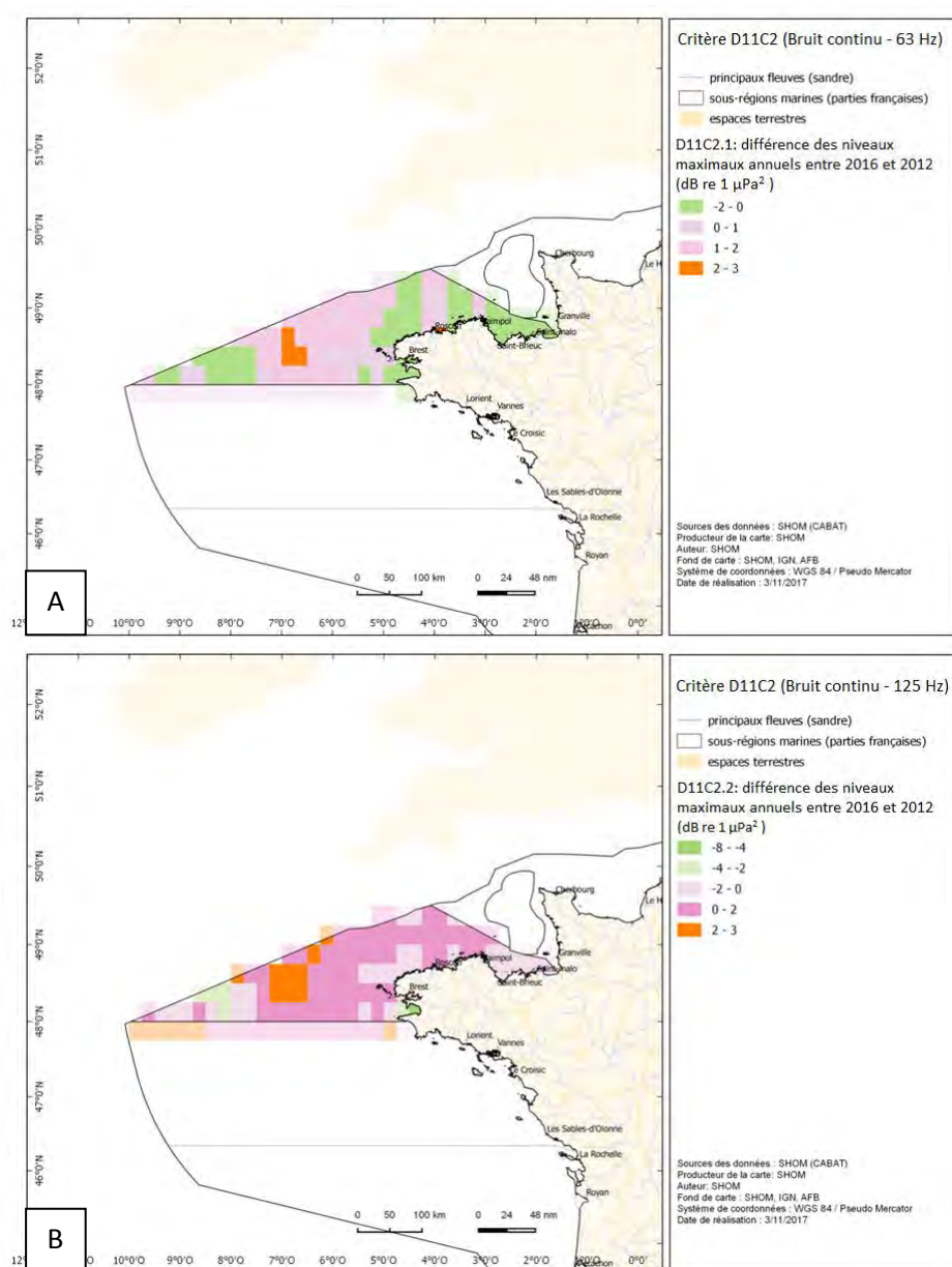
Figure 7 : Distribution spatiale de la différence des niveaux maximaux annuels entre 2016 et 2012 pour la bande de tiers d'octave centrée sur 63 Hz (A) et 125 Hz (B) dans la SRM MC.
