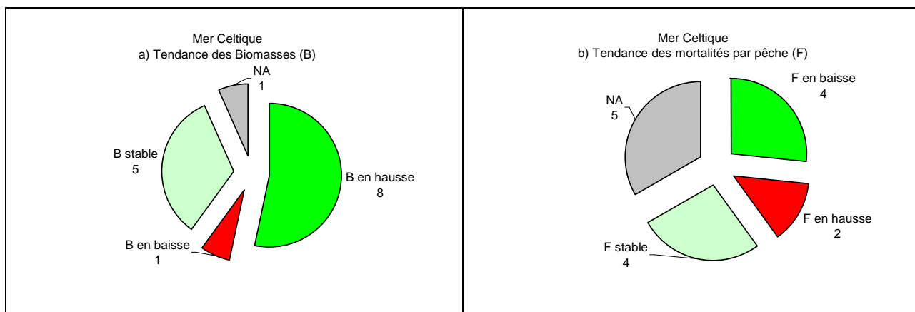
7 8 9 Figure 37 : Evolution des principaux stocks exploités (15) par les pêcheries françaises dans la sous-région marine mers Celtiques en 2010.
