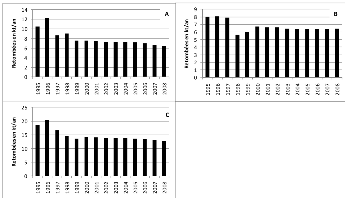
9 10 Figure 26 : Evolution inter-annuelle des retombées atmosphériques en azote oxydé (A), azote réduit (B) et azote total (C) de 1995 à 11 2008, en mers Celtiques, exprimées en kt d'azote par an.
