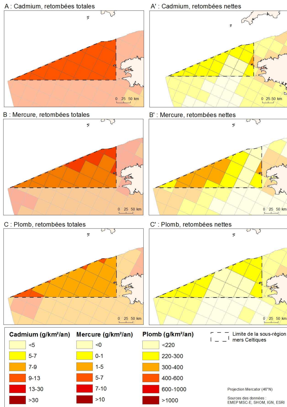
4 5 Figure 15 : Retombées atmosphériques totales et nettes en cadmium (A et A'), mercure (B et B') et plomb (C et C') en mers Celtiques 6 en 2008, exprimées en g/km2, selon le modèle EMEP.
