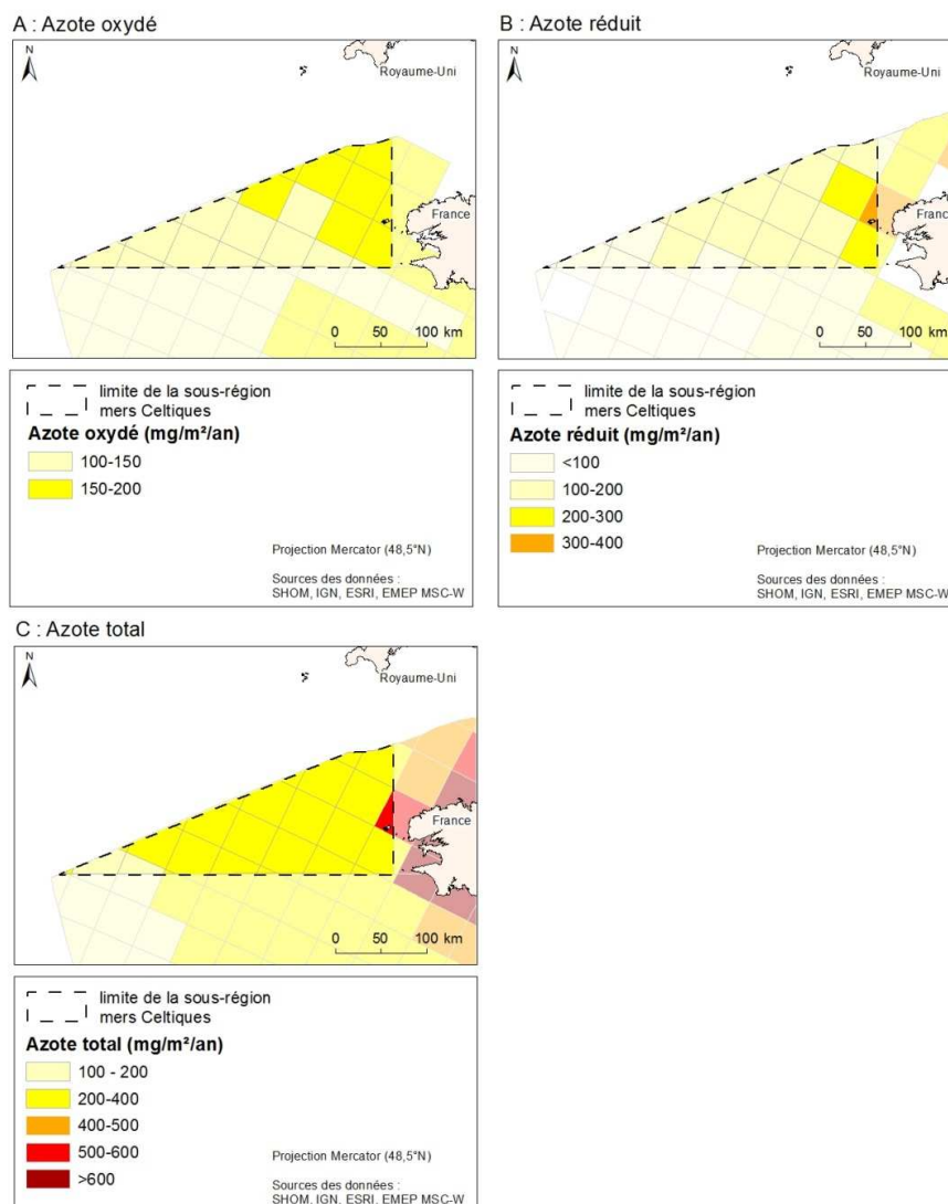
1 2 3 Figure 25 : Retombées atmosphériques en azote oxydé (A), azote réduit (B) et azote total (C) en mers Celtiques en 2008, exprimées en mg/m 2 , selon le modèle EMEP.
