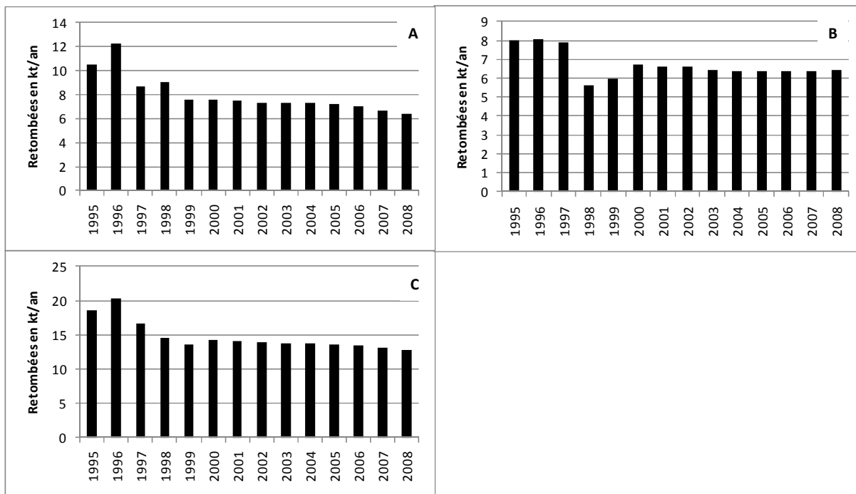
9 10 11 Figure 26 : Evolution inter-annuelle des retombées atmosphériques en azote oxydé (A), azote réduit (B) et azote total (C) de 1995 à 2008, en mers Celtiques, exprimées en kt d'azote par an.
