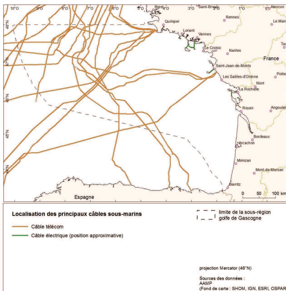
Figure 15 : Localisation des principaux câbles sous-marins dans la sous-région marine golfe de Gascogne. Source : AAMP.
